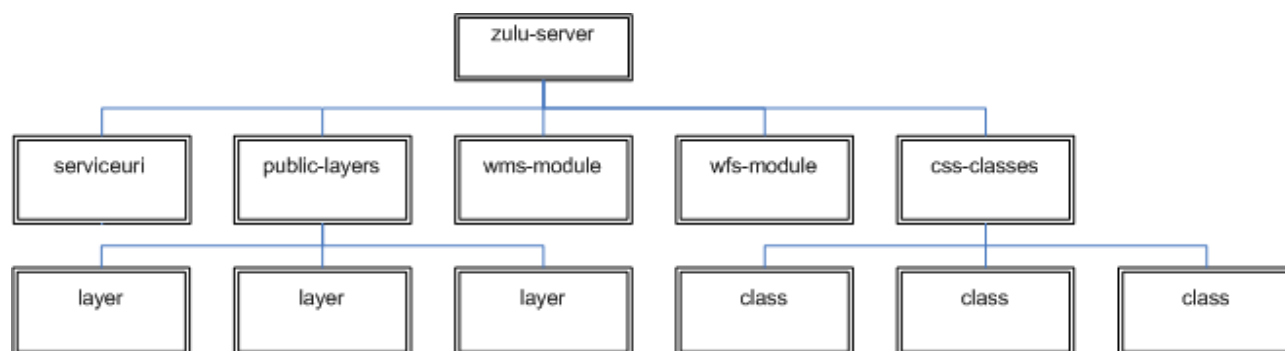
Рисунок 7.1 - Структура wms.xml
